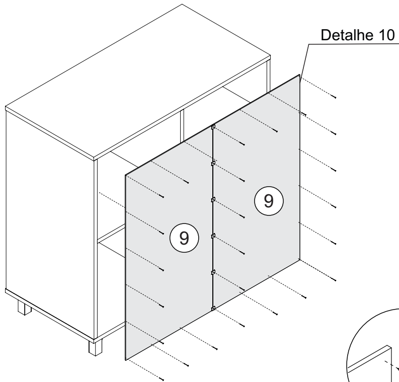
Detalhe 10 Detail/Detalle
