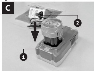
Figura C 1. Indicador de carga 2. Enchufe del cargador
