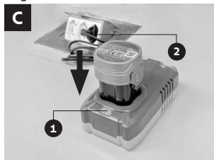
Figura C 1. Indicador de Carga 2. Plugue do carregador
